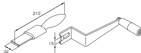
●ハブボルトにハンドルをセットし、ディスクローターを回しながら行います。
