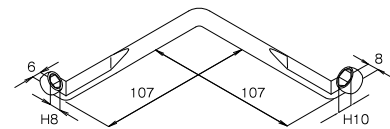
ケース外形寸法 W200×L90×H25 / 0.142kg
