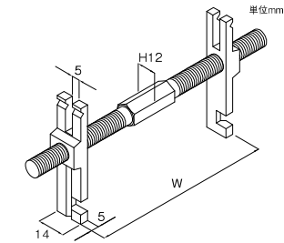
●ライニングを広げてシリンダー交換に
